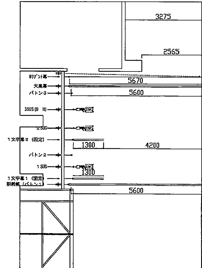
【 断面図 】
